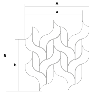
A 34,2 cm - 13 1 / 2 " a 30,5 cm - 12" B 38 cm - 15" b 27,7 cm - 10 7 / 8 "
